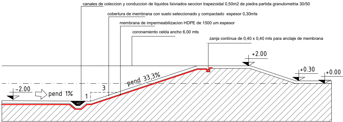
DETALLE DRENES y MEMBRANA Ecoparque Gualaguaychu
