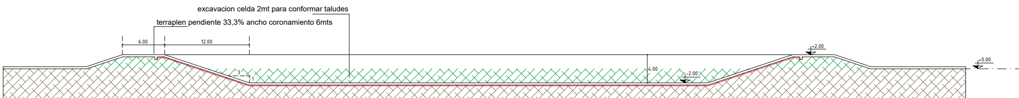
CORTE A-A Ecoparque Gualaguaychu
