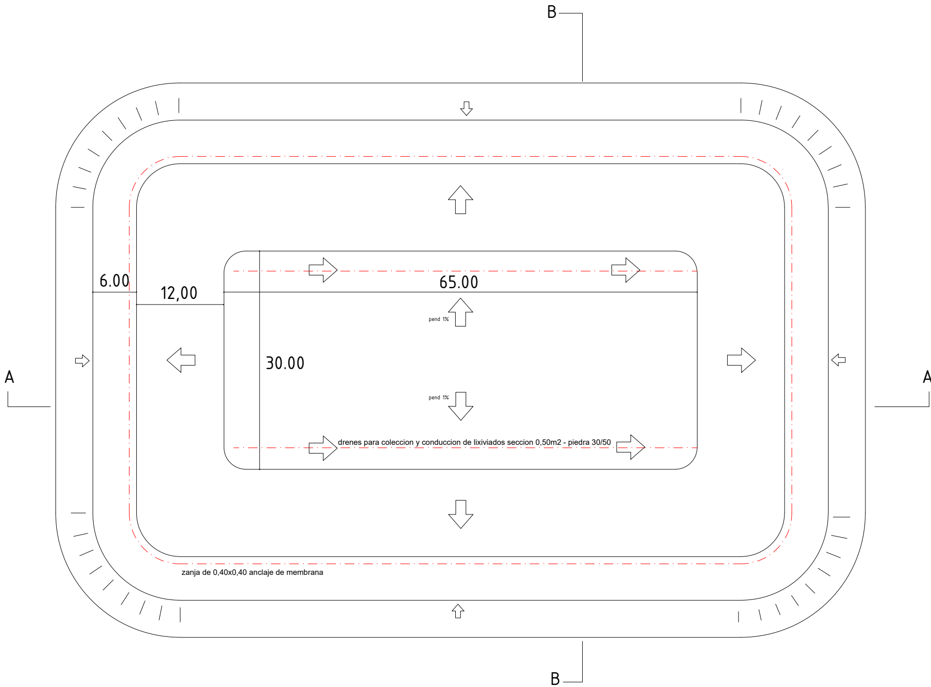
PLANTA CELDA Ecoparque Gualaguaychu
