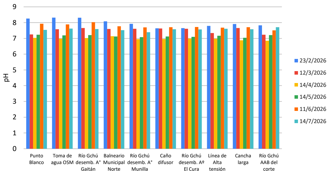
Río Gualagaychú (febrero a julio 2026) - pH
