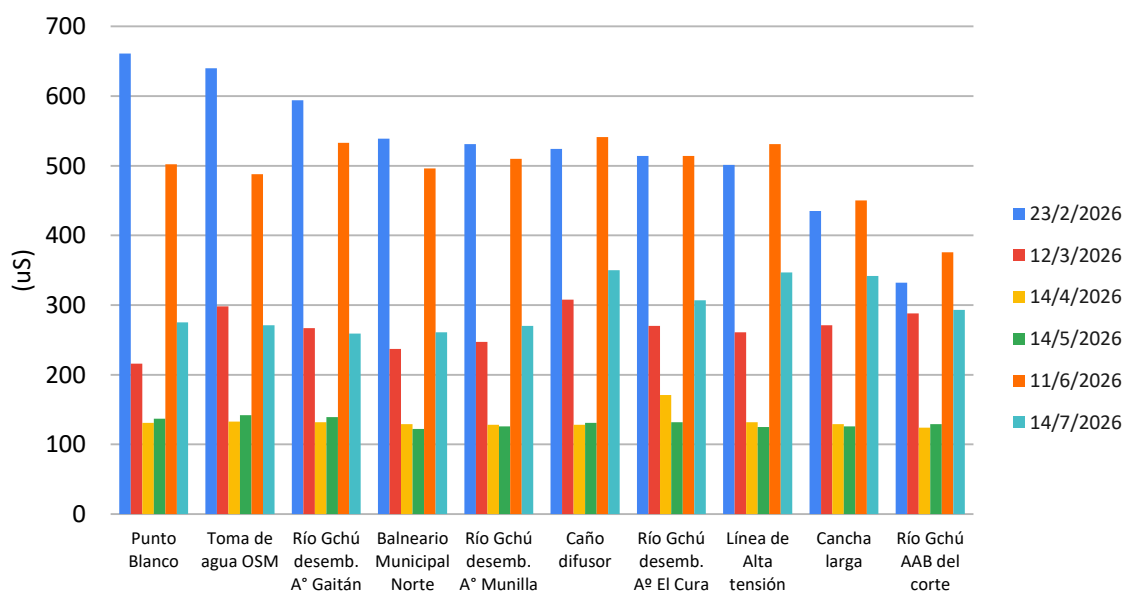
Río Gualagaychú (febrero a julio 2026) - Conductividad
