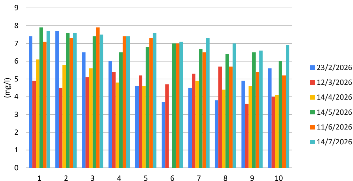
Río Gualagaychú (febrero a julio 2026) - Oxígeno Disuelto
