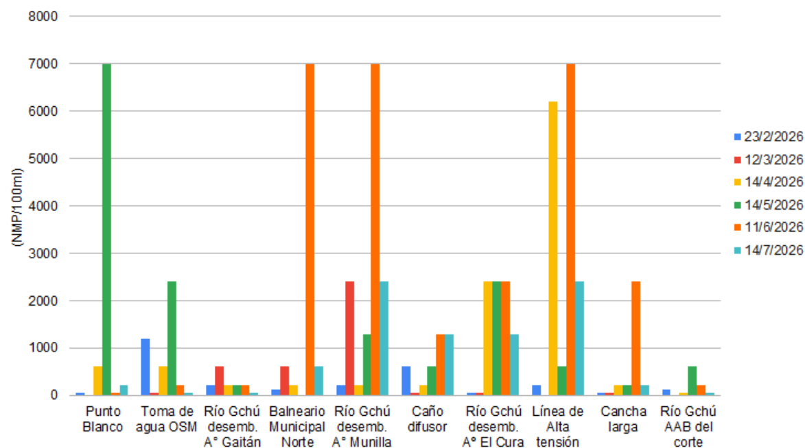
Río Gualagaychú (febrero a julio 2026) - Coliformes Fecales
