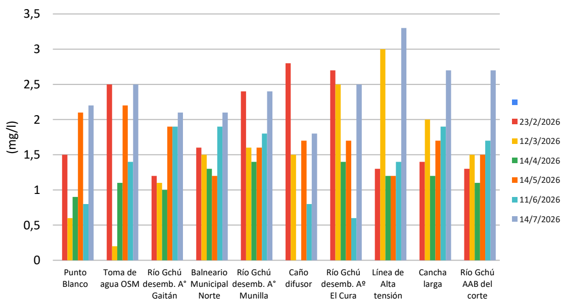
Río Gualagaychú (febrero a julio 2026) - Demanda Biológica de Oxígeno
