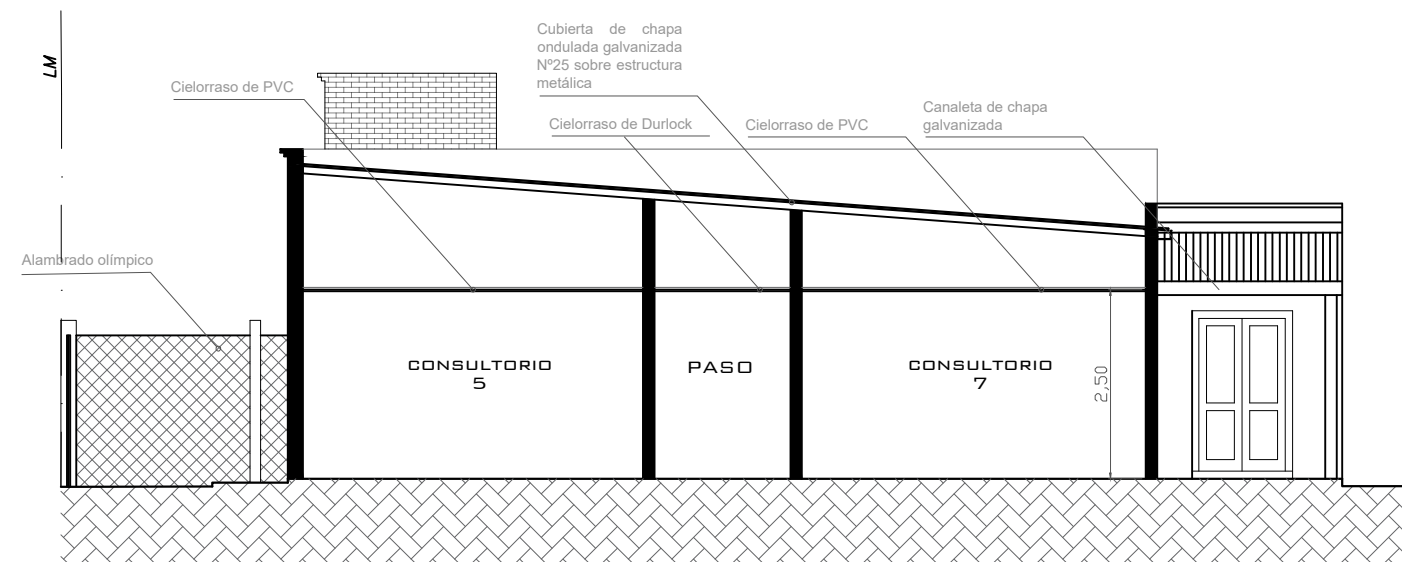
Corte B-B
