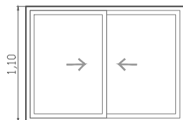
V1 - CONSULTORIOS / SUM
